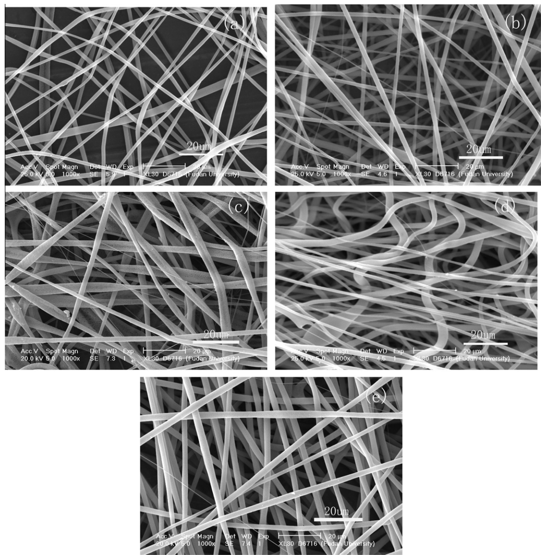
Fig. 4. SEM micrographs of the products: (a) F1 fiber, (b) F2 fiber, (c) F3 fiber, (d) F4 fiber, (e) PLLA fiber.
